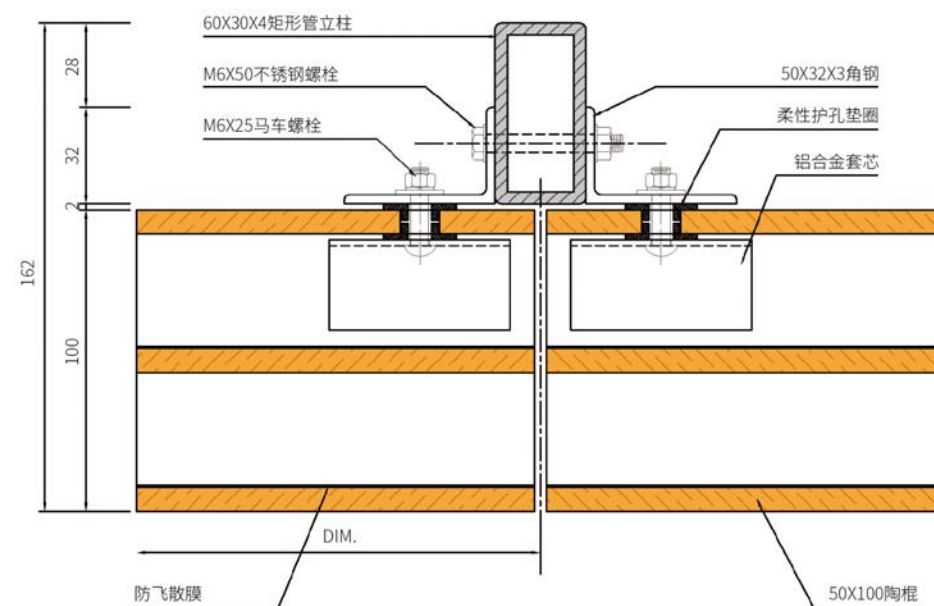
陶棍横剖节点图
