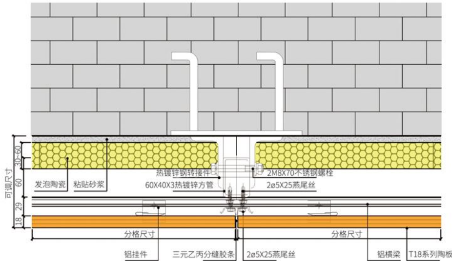
T18横剖节点图
