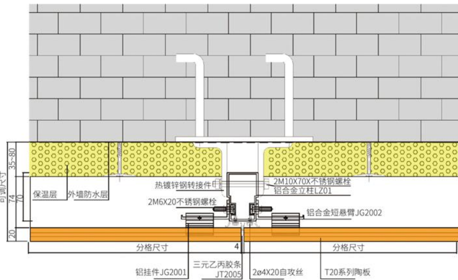
T20横剖节点图
