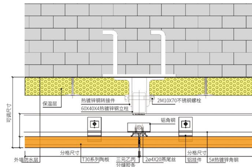
T30横剖节点图
